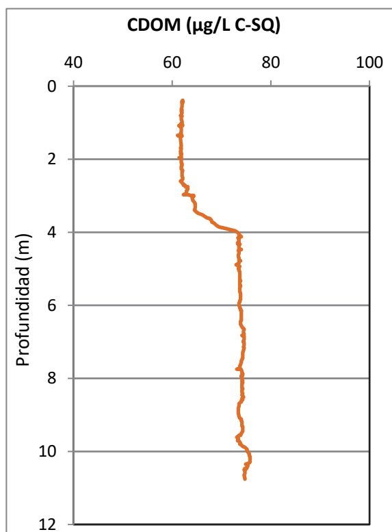
Figura 5. Perfil vertical de la conductividad y la materia orgánica cromofórica.
