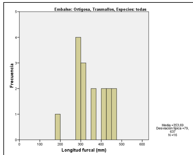
Figura 17: Frecuencia de tallas para todas las especies capturadas en Ortigosa.
