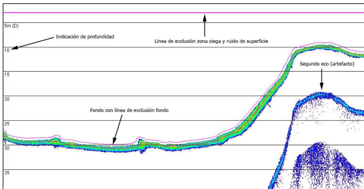
Figura 18: Ecograma prospección vertical, embalse de Ortigosa. Destaca la ausencia de señales en la columna de agua. Umbral TS -60 dB, correspondiente a peces menores de 1,7 cm de talla.
