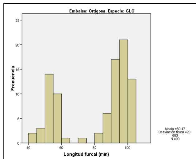
Figura 13: Frecuencia de tallas para Gobio lozanoi .
