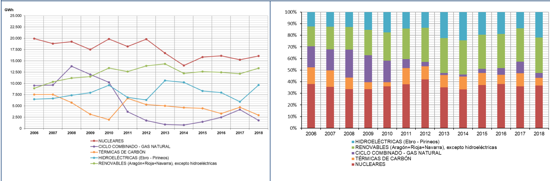
Figura 25. Evolución de la producción eléctrica anual en la demarcación hidrográfica del Ebro por fuentes (GWh) (2006-2018)
