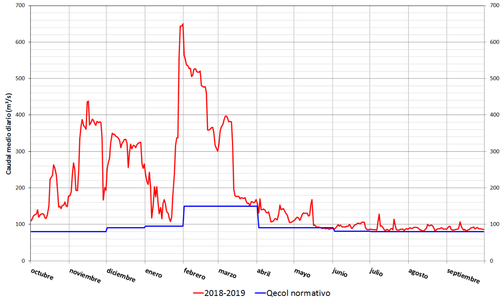
Figura 35. Hidrograma de la estación de aforos 027 Ebro en Tortosa año 2018-19 (caudales medios diarios) y el régimen de caudales ecológicos mínimos establecido en el Plan Hidrológico 2015-2021 (m 3 /s)
