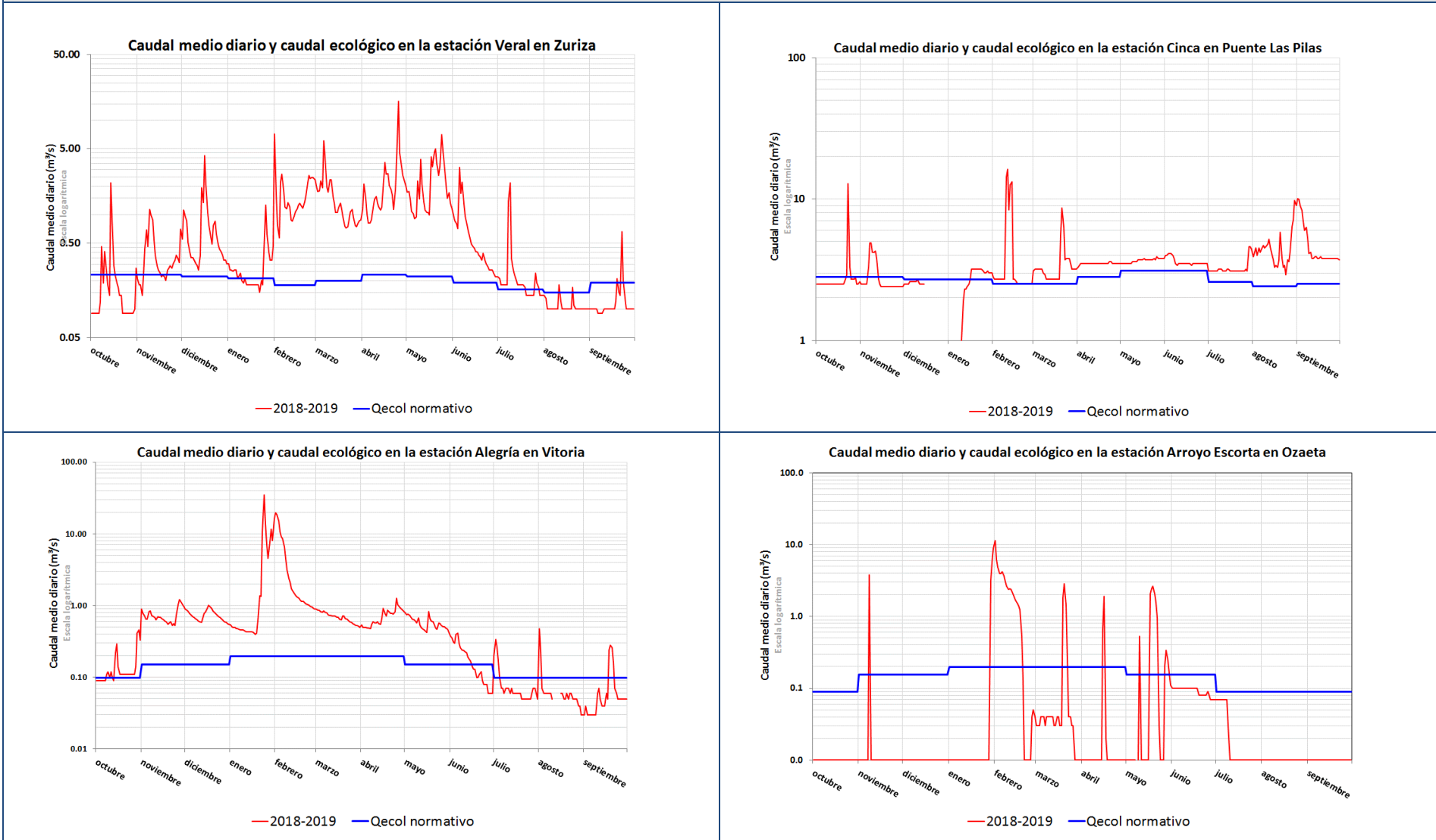
Figura 34. Incumplimientos de regímenes de caudales ecológicos y detalle en caudales bajos.
