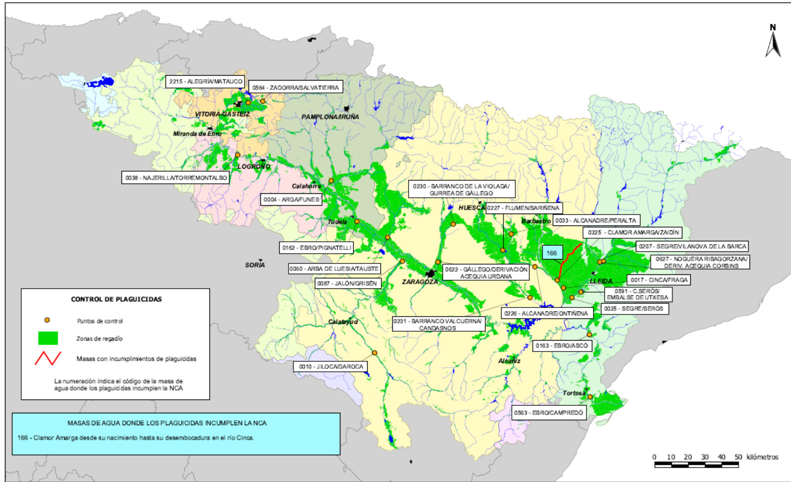
Figura 33. Control de plaguicidas (2018)
