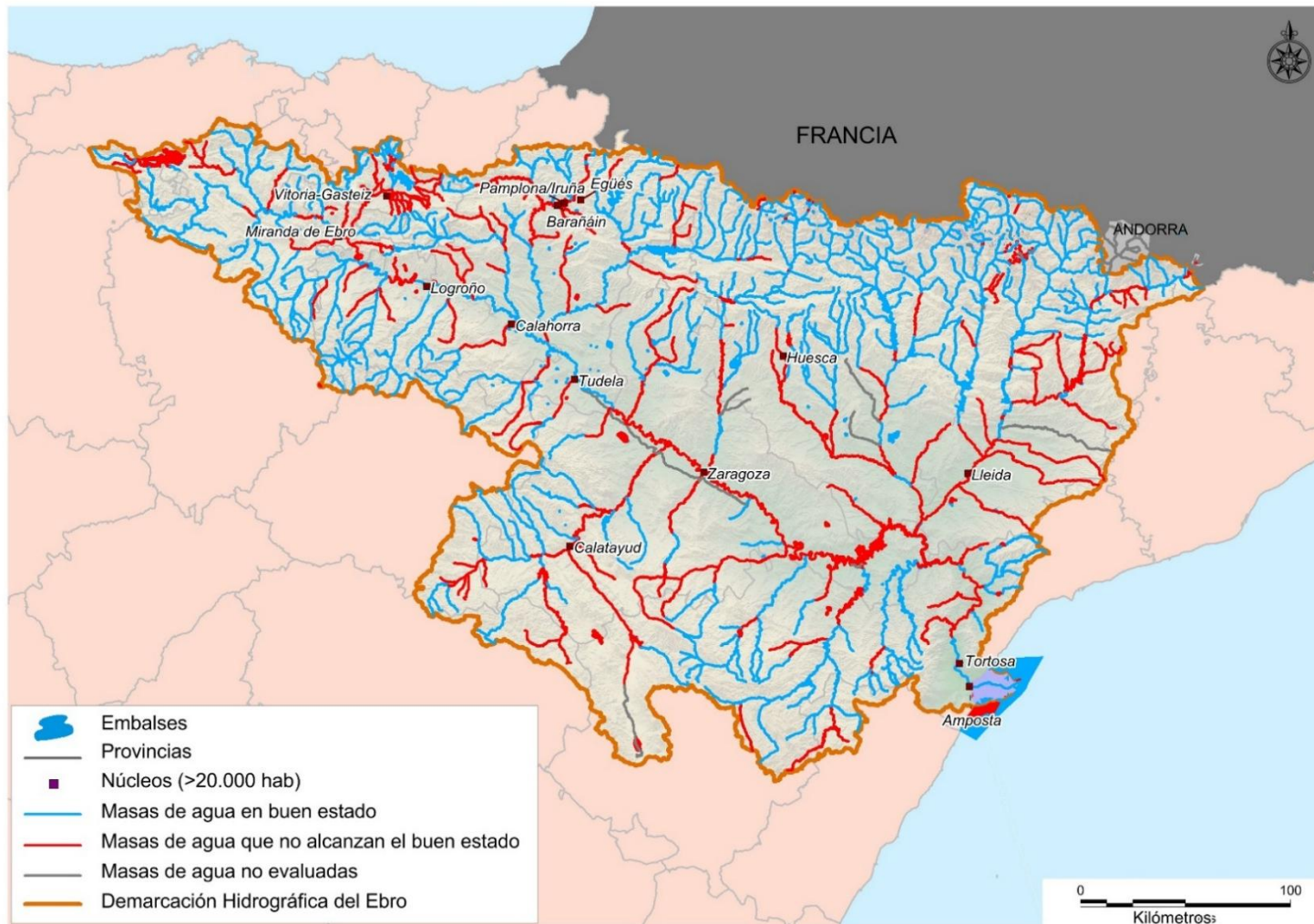
Figura 36. Estado de las masas de agua superficial (MASp) en la demarcación del Ebro (PHE 2015-2021)
