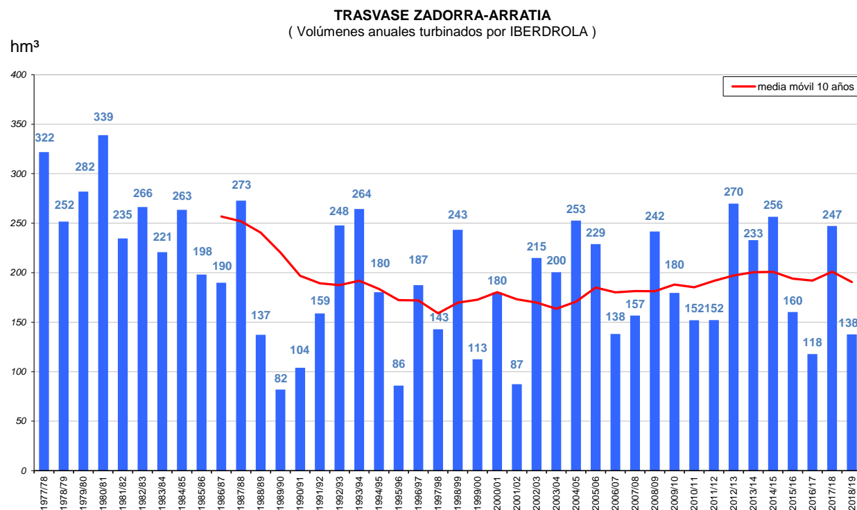
Figura 27. Evolución anual de los volúmenes transferidos fuera la demarcación hidrográfica del Ebro (trasvases principales no reversibles). Traslase Zadorra-Arratia (Gran Bilbao)
