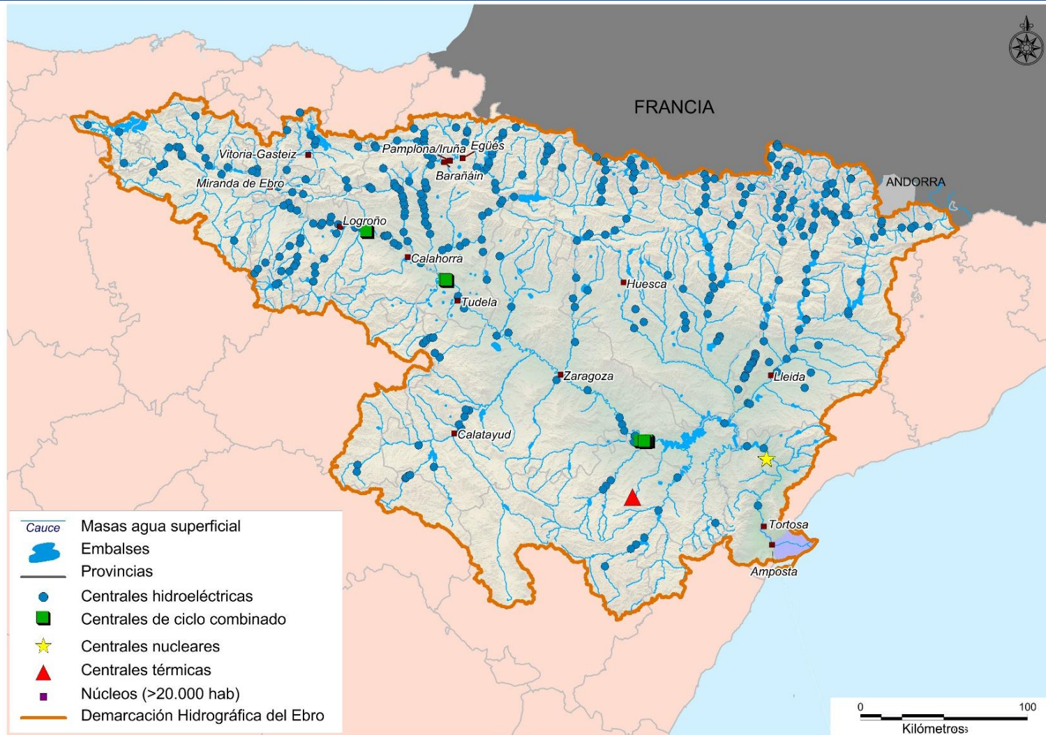
Figura 26. Localización de las principales centrales de producción eléctrica
