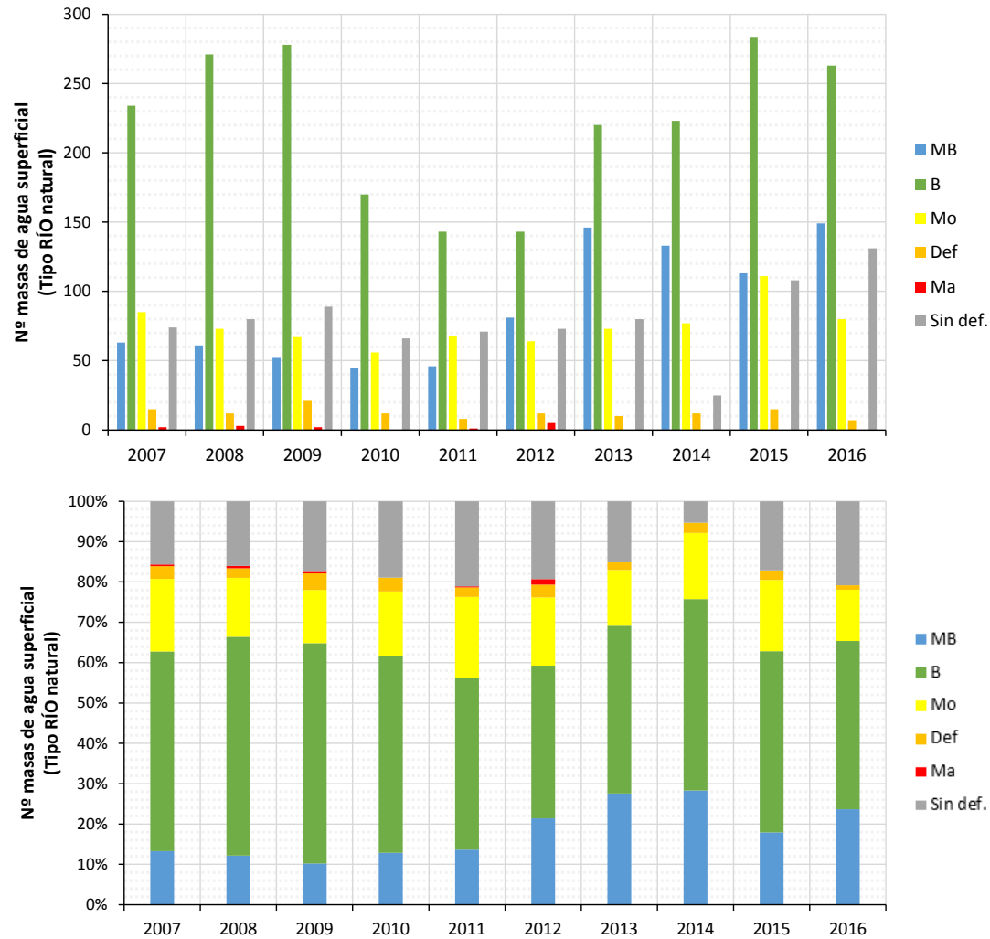
Figura 37. Masas de agua superficial (MASp) tipo RÍO
