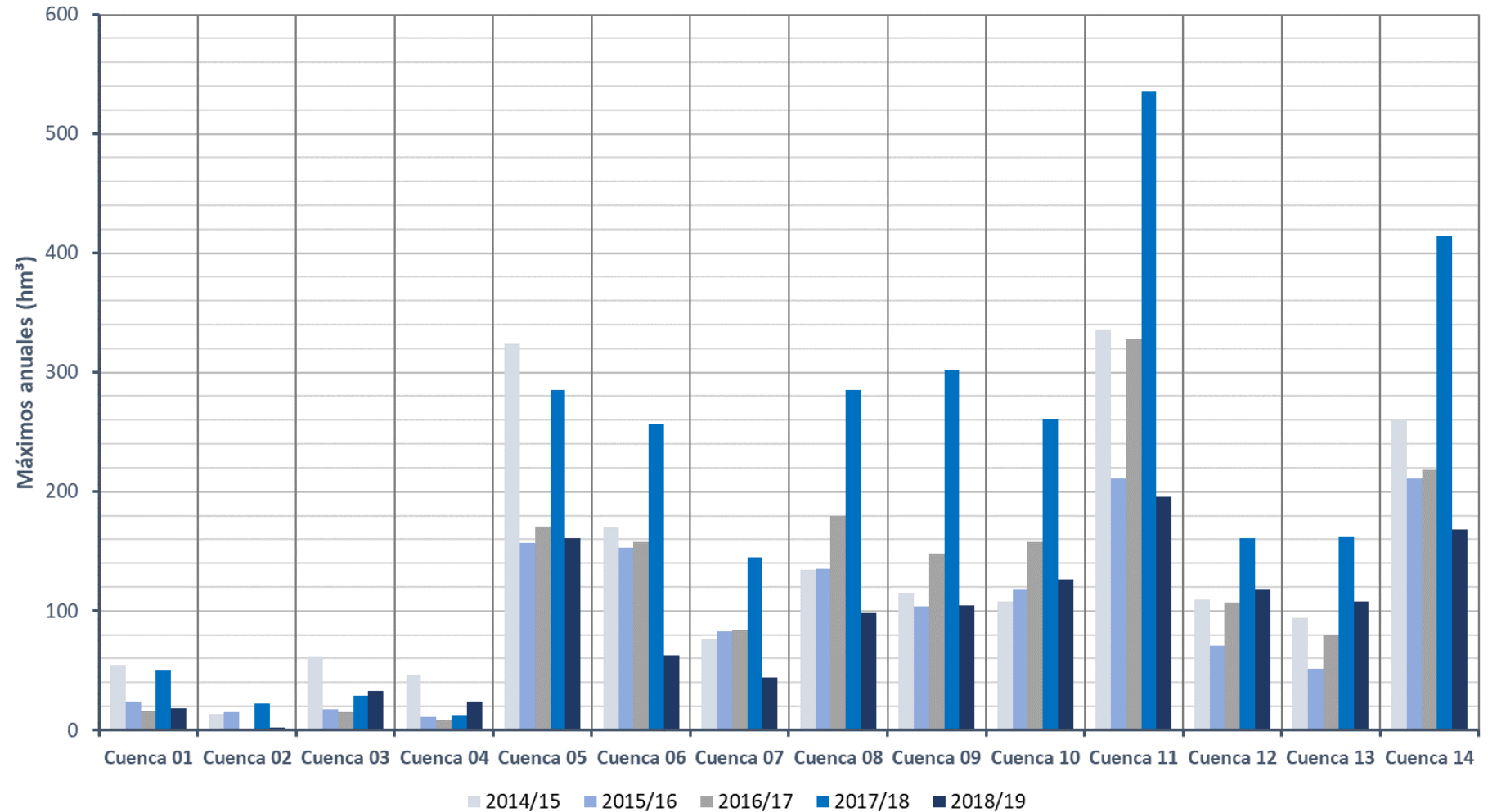
Figura 15. Distribución de la medición máxima en el año para el recurso nieve en las 14 cuencas nivales de la DHE (2014-2019)
