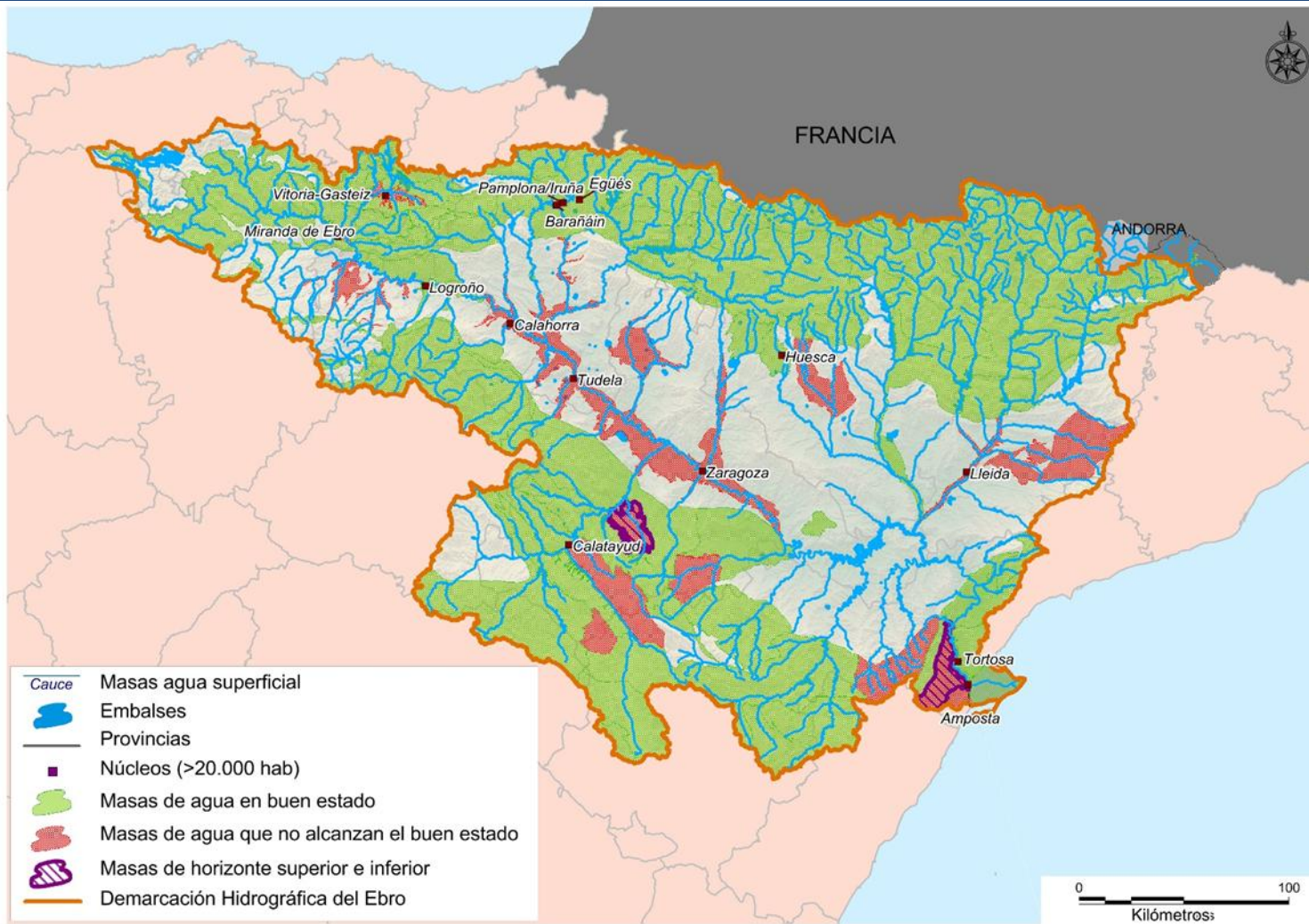
Figura 38. Estado de las masas de agua subterránea (MASb) en la demarcación del Ebro (PHE 2015-2021)
