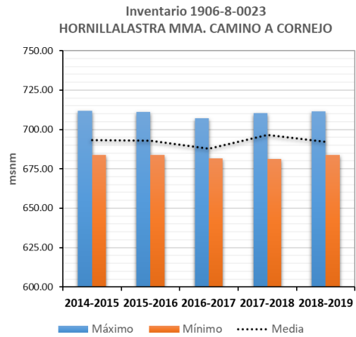
Figura 17. Evolución de la piezometría (2014-2019)
